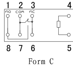
接线图
