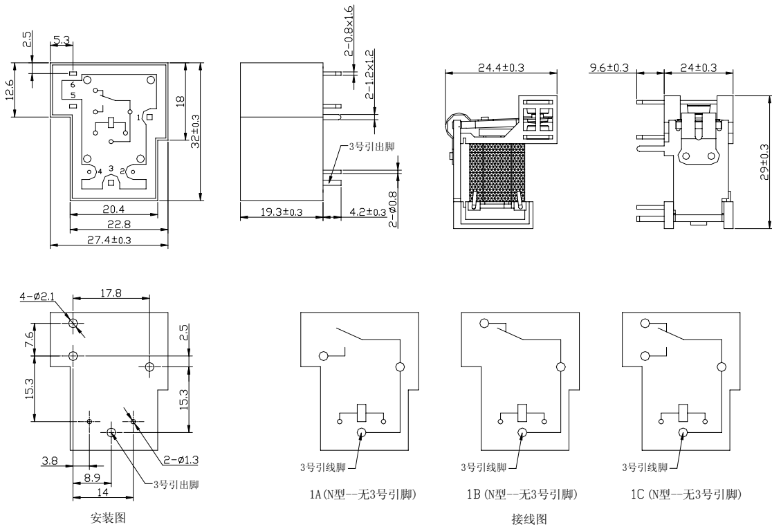
安装图
